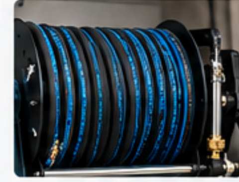
ÇİFT HORTUM TAMBURU 60 m x 1/2" + 60 m x 3/8".
